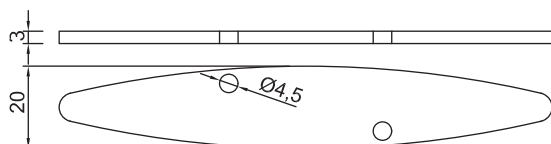
SL-82 GM-NEWZ-06 End Cap
