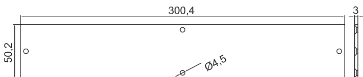
SL-158 GM-NEWZ-131 End Cap
