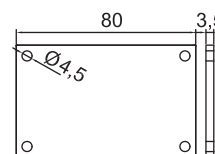
SL-125 GM-NEWZ-97 End Cap
