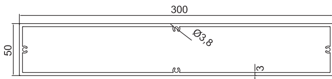
SL-181 GM-NEWZ-101 End Cap
