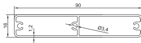
GM-NEWZ-09 90x16mm Louvre Blade 0.86kg/m
