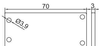
SL-17 GM-NEWZ-52 End Cap
