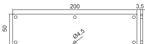
SL-181 GM-NEWZ-101 End Cap
