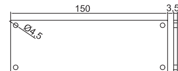
SL-126 GM-NEWZ-98 End Cap
