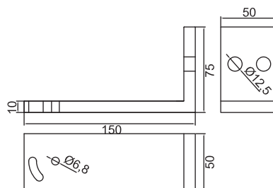
SL-155 GM-NEWZ-157 150mm Stand
