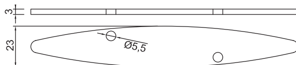
SL-182 GM-NEWZ-70 End Cap
