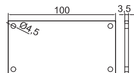
SL-152 GM-NEWZ-120 End Cap
