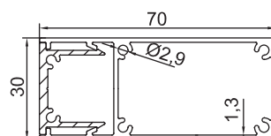
GM-NEWZ-52&53 30x70mm Louvre Blade 1.22kg/m
