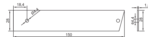
GM-NEWZ-181 End Cap 0.011kg/m
