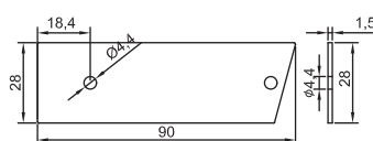
GM-NEWZ-181 End Cap 0.011kg/m
