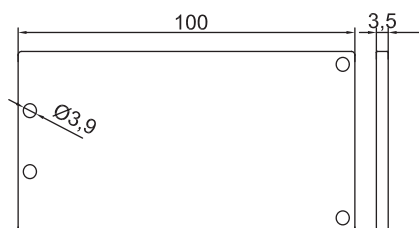
SL-15 GM-NEWZ-55 End Cap
