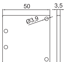
SL-16 GM-NEWZ-54 End Cap
