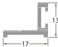
GM-NEWZ-W29 Door Stopper 0.100 kg/m
