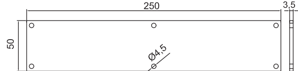
SL-180 GM-NEWZ-100 End Cap
