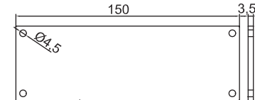
SL-126 GM-NEWZ-98 End Cap
