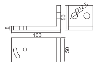
SL-156 GM-NEWZ-157 100mm Stand
