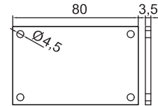
SL-125 GM-NEWZ-97 End Cap
