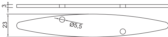
SL-182 GM-NEWZ-70 End Cap
