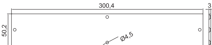
SL-158 GM-NEWZ-131 End Cap
