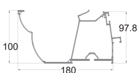
GM-NEWZ-Y13063 A5 - Straight Edge Gutter
