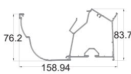
GM-NEWZ-Y13012 A3 - Radius Edge Gutter
