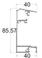
GM-NEWZ-Y13059 A5 - Wall Edge
