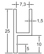
GM-NEWZ-151 Mesh Frame 0.217 kg/m
