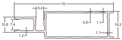
GM-NEWZ-W25 Door Frame 0.528 kg/m
