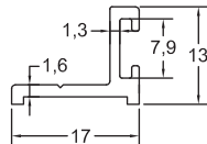
GM-NEWZ-W29 Door Stopper 0.100 kg/m
