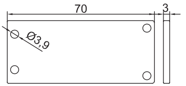
SL-17 GM-NEWZ-52 End Cap
