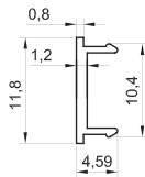
GM-NEWZ-183 181 / 182 Side Cap 0.05kg/m
