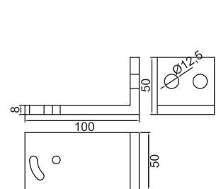
SL-156 GM-NEWZ-157 100mm Stand
