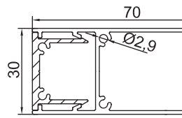
GM-NEWZ-52&53 30x70mm Louvre Blade 1.22kg/m
