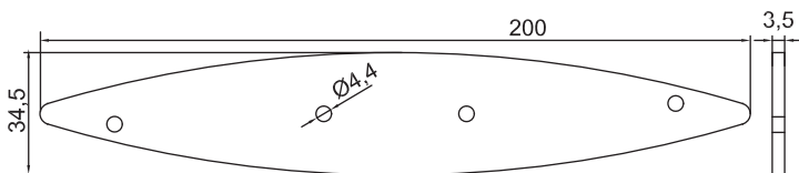
SL-165 GM-NEWZ-102 End Cap
