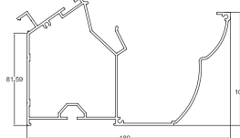
GM-NEWZ-Y13064 A5 Radius Edge Gutter
