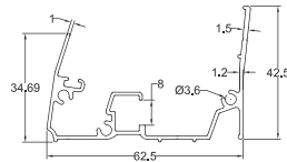
GM-NEWZ-Y13007 Wall Edge
